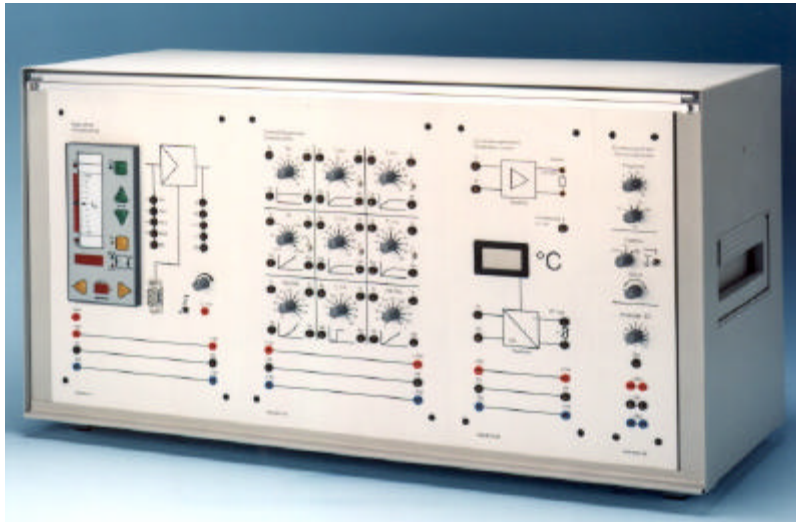
Regelmodell SIPART DR20 mit Regelstrecken-Simulatoren
